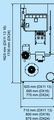
Rückansicht DX 11 13 16 24
