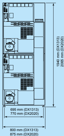
Seitenansicht DX 13/13 20/20
