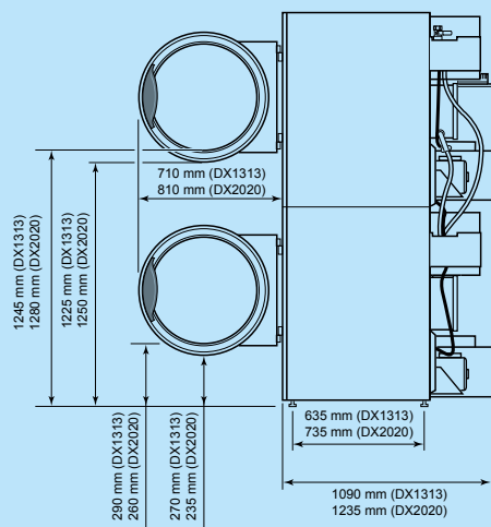
Seitenansicht DX 13/13 20/20
